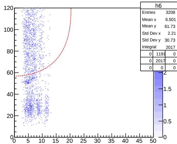
Etot[5]:ThetaLab[5] {tgtc&lt;8.0&amp;&amp;DetectorNumber[5]==6}
