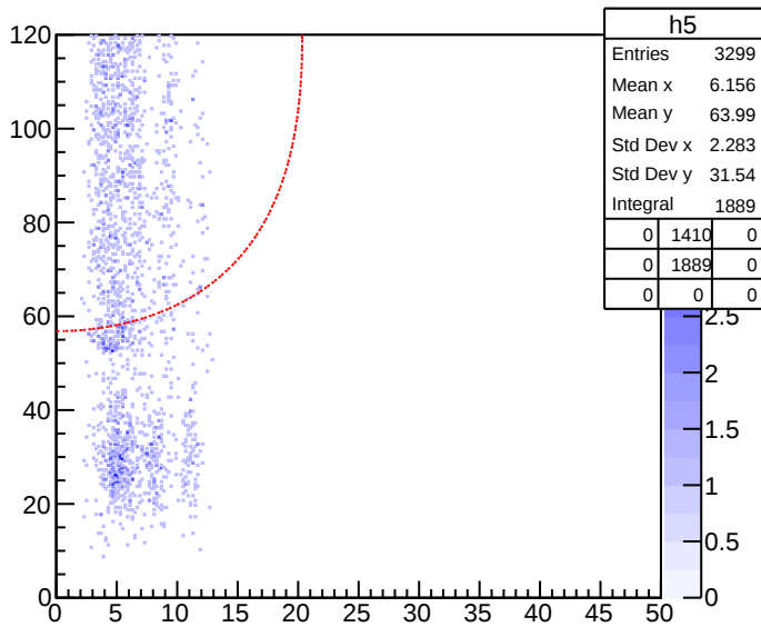
Etot[5]:ThetaLab[5] {tgtc&lt;8.0&amp;&amp;DetectorNumber[5]==5}
