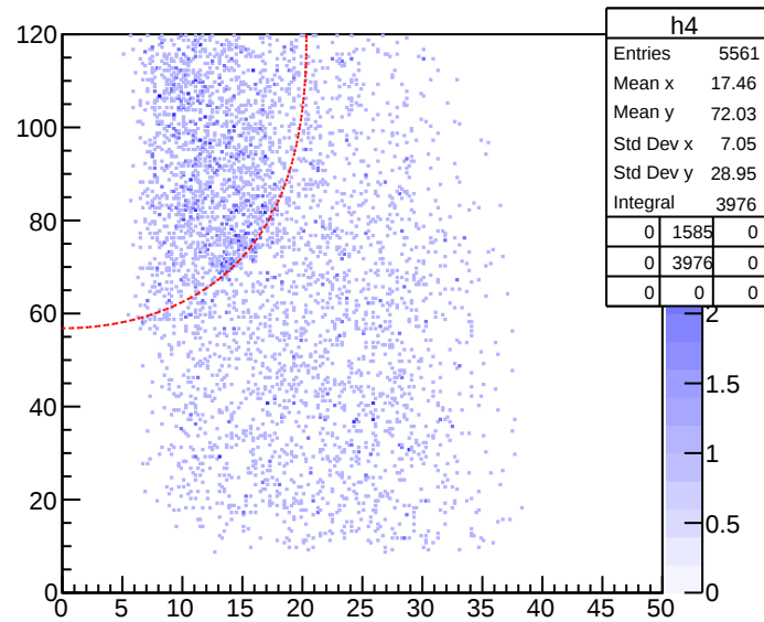
Etot[5]:ThetaLab[5] {tgtc&lt;8.0&amp;&amp;DetectorNumber[5]==4}
