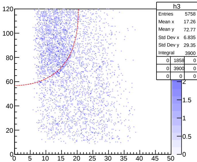
Etot[5]:ThetaLab[5] {tgtc&lt;8.0&amp;&amp;DetectorNumber[5]==3}
