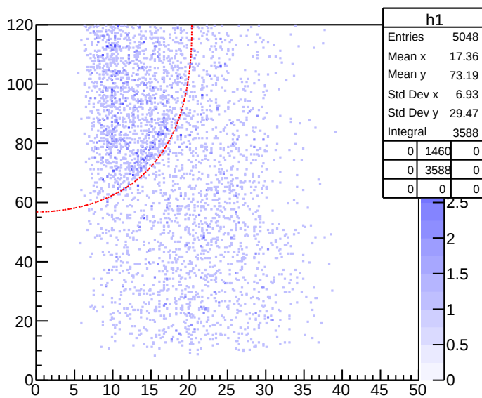
Etot[5]:ThetaLab[5] {tgtc&lt;8.0&amp;&amp;DetectorNumber[5]==1}
