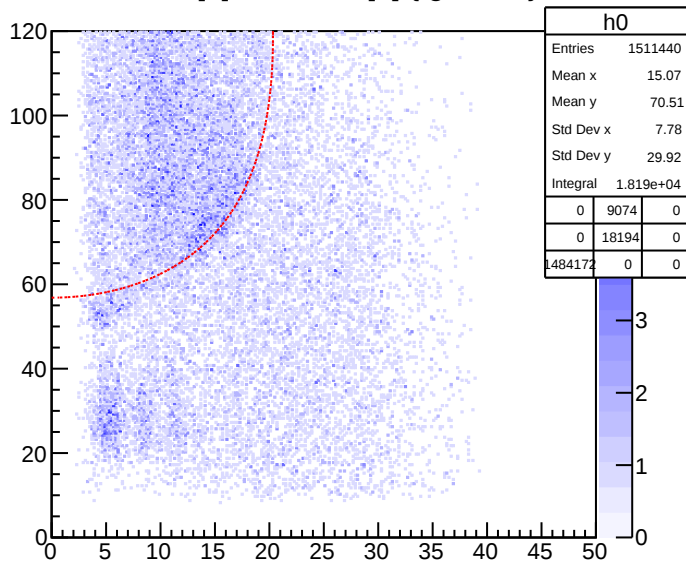
Etot[5]:ThetaLab[5] {tgtc&lt;8.0}
