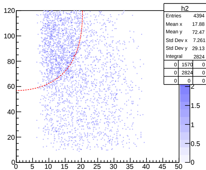
Etot[5]:ThetaLab[5] {tgtc&lt;8.0&amp;&amp;DetectorNumber[5]==2}
