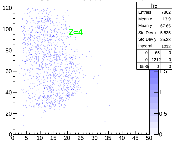
Etot[4]:ThetaLab[4] {tgtc&lt;8.0&amp;&amp;z4}
