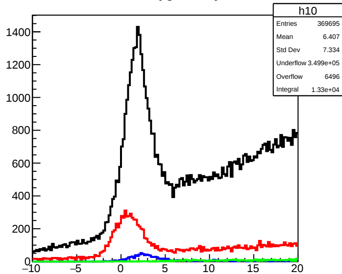
Exd {tgtc&lt;8.0}
