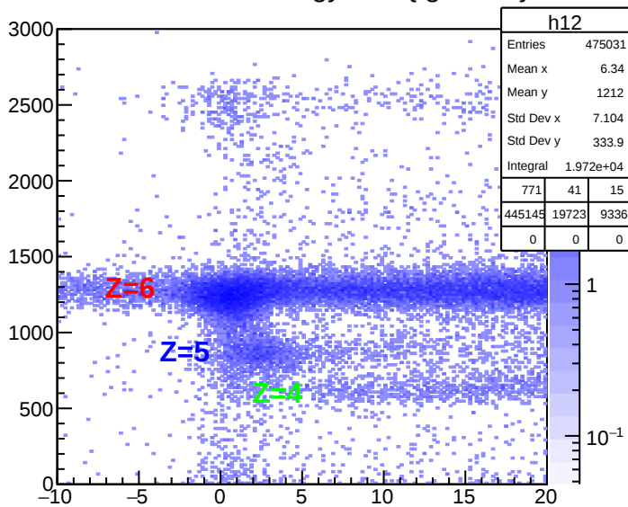
ICNumexo.Energy:Exd {tgtc&lt;8.0}
