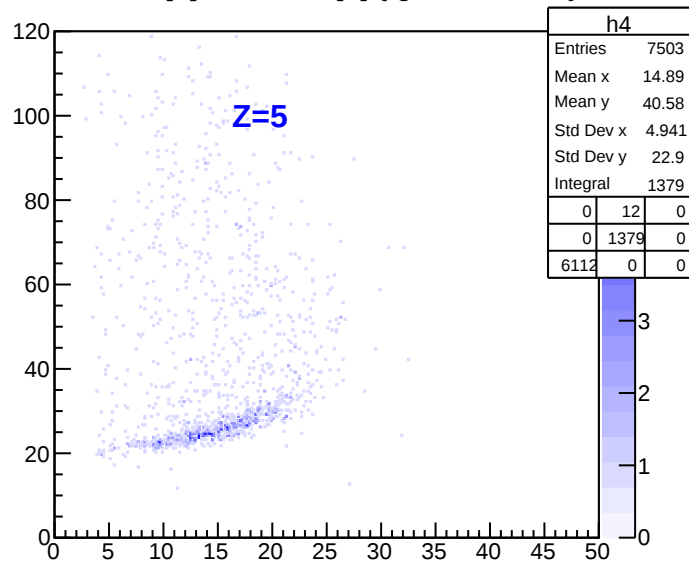
Etot[4]:ThetaLab[4] {tgtc&lt;8.0&amp;&amp;z5}
