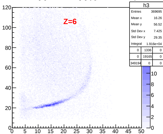
Etot[4]:ThetaLab[4] {tgtc&lt;8.0&amp;&amp;z6}
