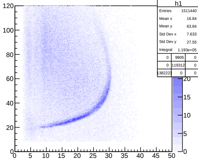
Etot[4]:ThetaLab[4] {tgtc&lt;8.0}
