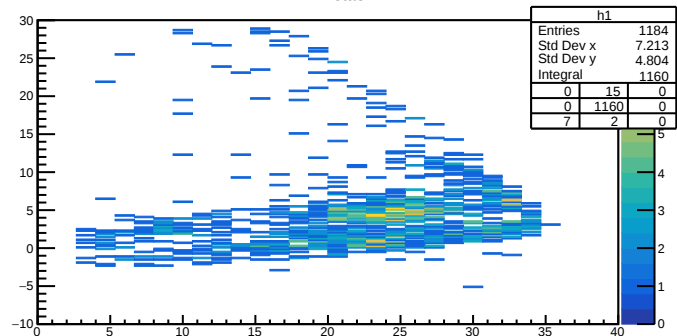
Ex:Theta3
