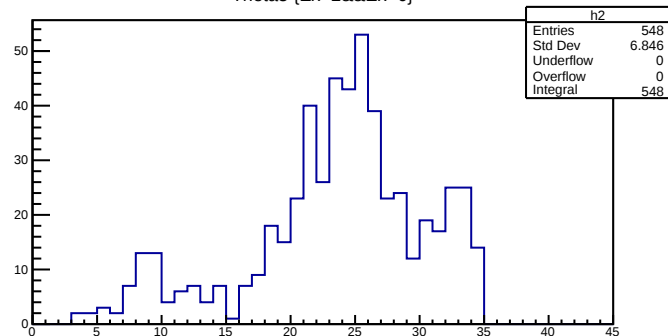
Theta3 {Ex&gt;2&amp;&amp;Ex&lt;6}
