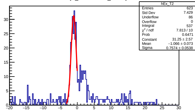
Ex {X_M2&lt;0 &amp;&amp; Y_M2&lt;0}
