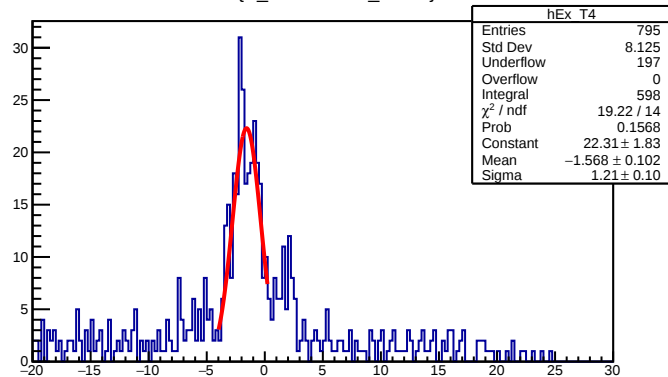
Ex {X_M2&gt;0 &amp;&amp; Y_M2&gt;0}
