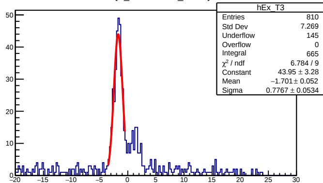
Ex {X_M2&gt;0 &amp;&amp; Y_M2&lt;0}
