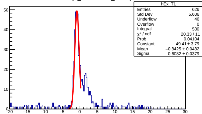
Ex {X_M2&lt;0 &amp;&amp; Y_M2&gt;0}
