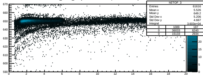
SI_TX:SI_EX {MUST2.TelescopeNumber==3}
