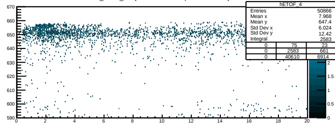
SI_TX:SI_EX {MUST2.TelescopeNumber==4}
