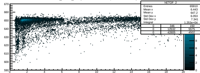
SI_TX:SI_EX {MUST2.TelescopeNumber==2}
