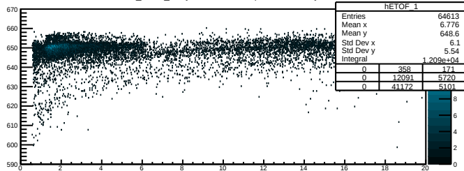
SI_TX:SI_EX {MUST2.TelescopeNumber==1}
