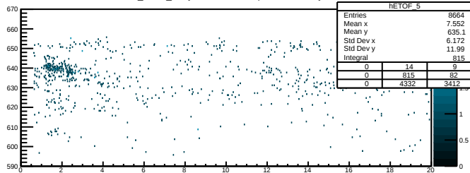
SI_TX:SI_EX {MUST2.TelescopeNumber==5}
