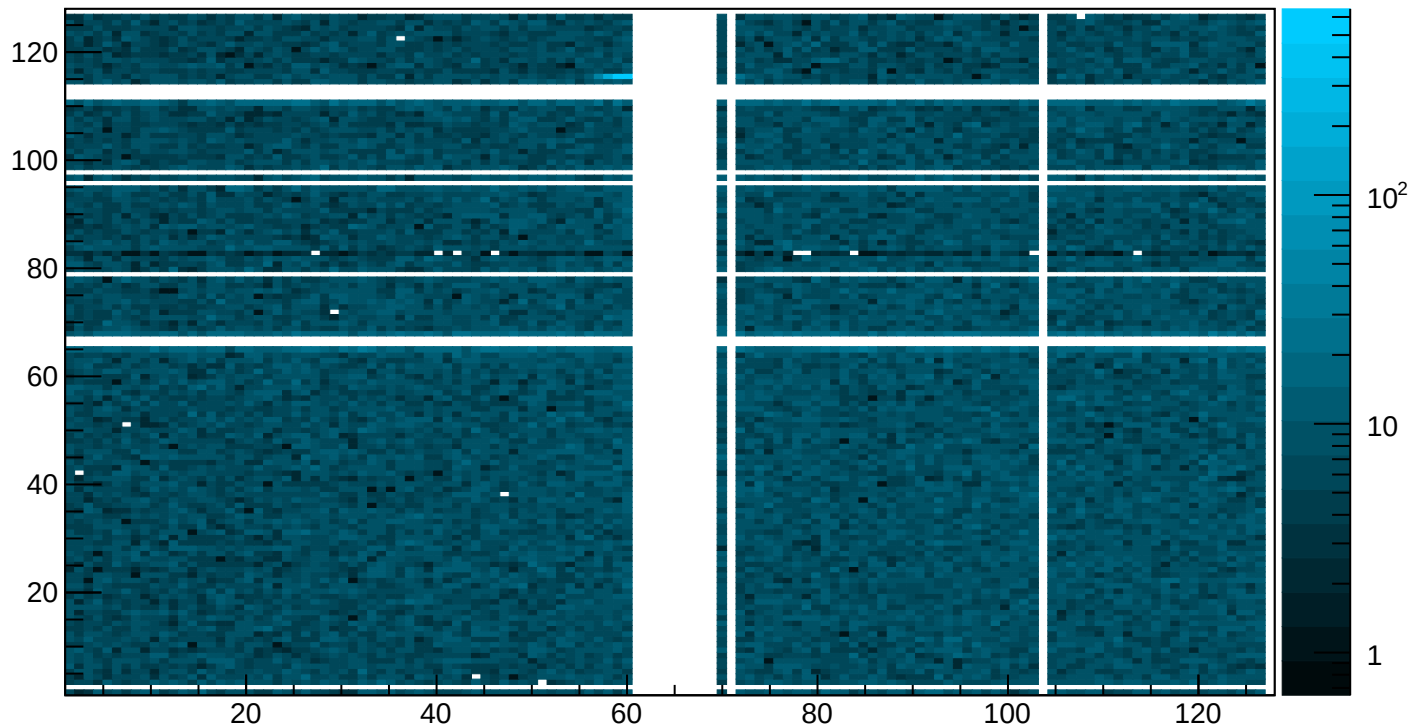
Si_Y:Si_X {TelescopeNumber==6}
