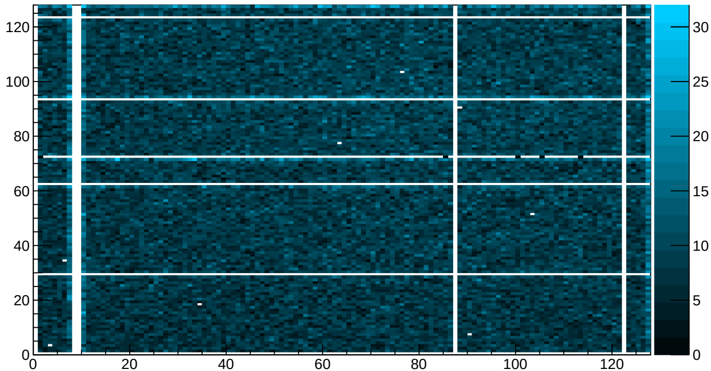
Si_Y:Si_X {TelescopeNumber==4}
