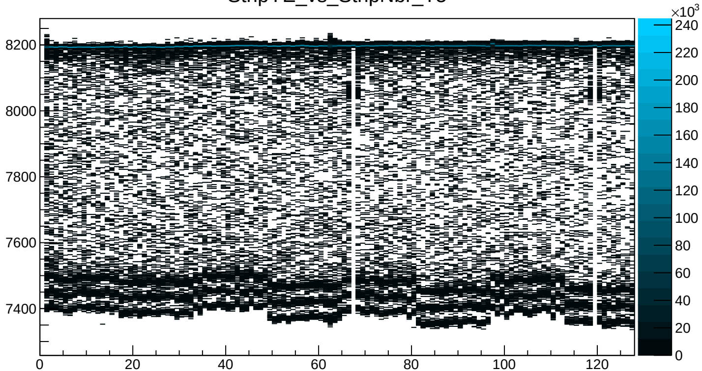
StripYE_vs_StripNbr_T5
