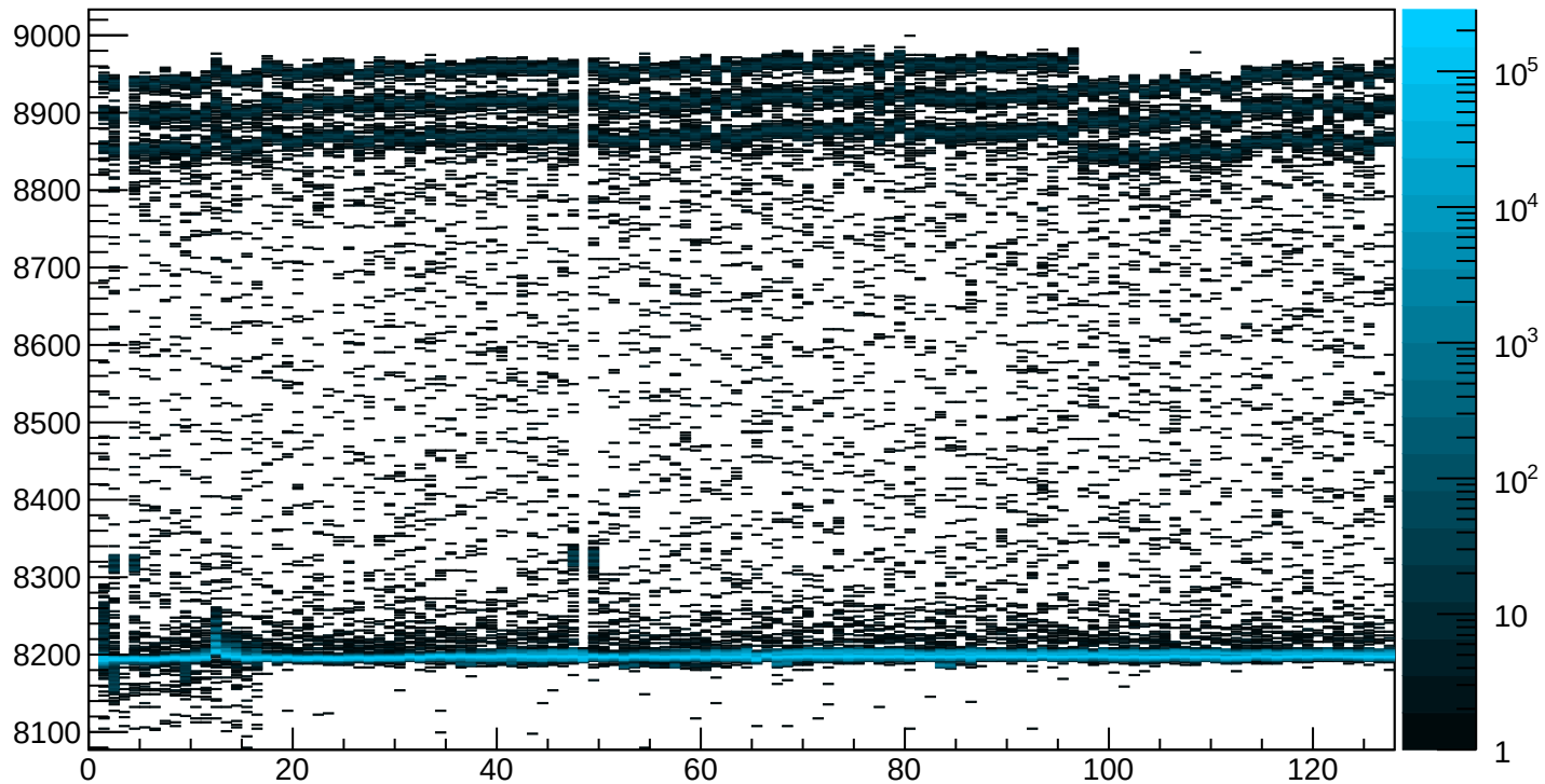
StripXE_vs_StripNbr_T5
