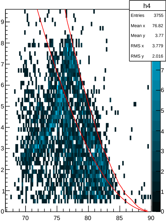
Si_E:ThetaLab {Csl_E<0&&GATCONF==32&&tar}
