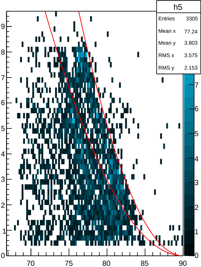
Si_E:ThetaLab {Csl_E<0&&GATCONF==64&&tar}
