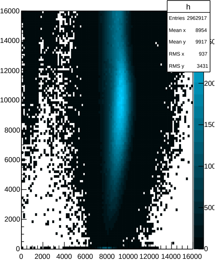
CHIO:QPlast {GATCONF==256}
