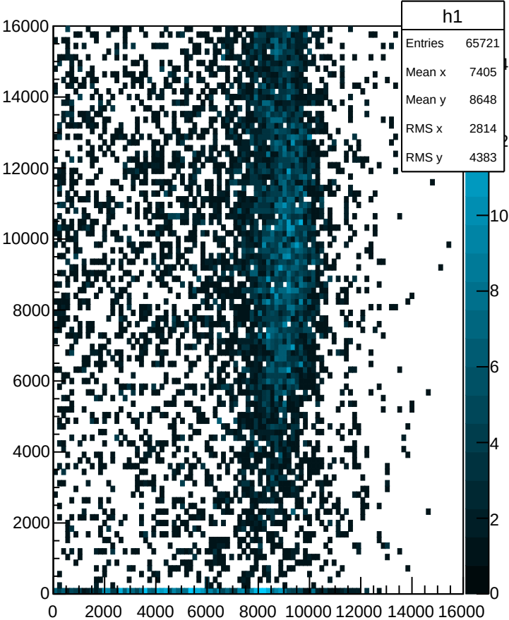
CHIO:QPlast {Csl_E<0&&GATCONF<16&&tar&&(m31||m34)}
