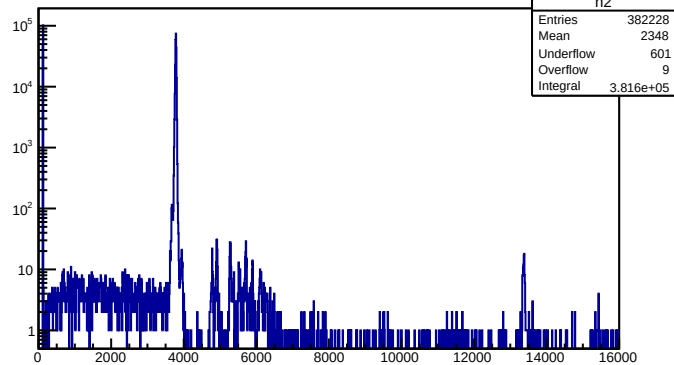
T_PLchCATS1
