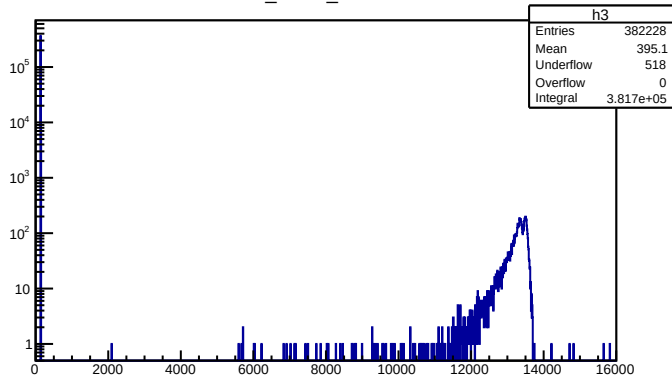
T_MUVI_CATS1
