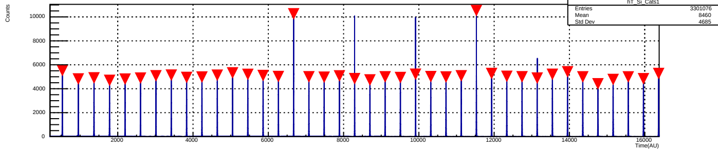
Histogram T_Si_Cats1
