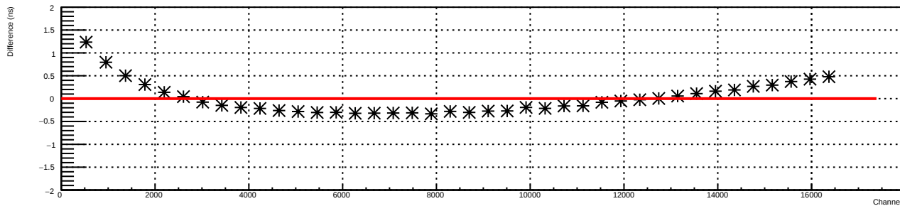
Histogram T_Si_Cats1
