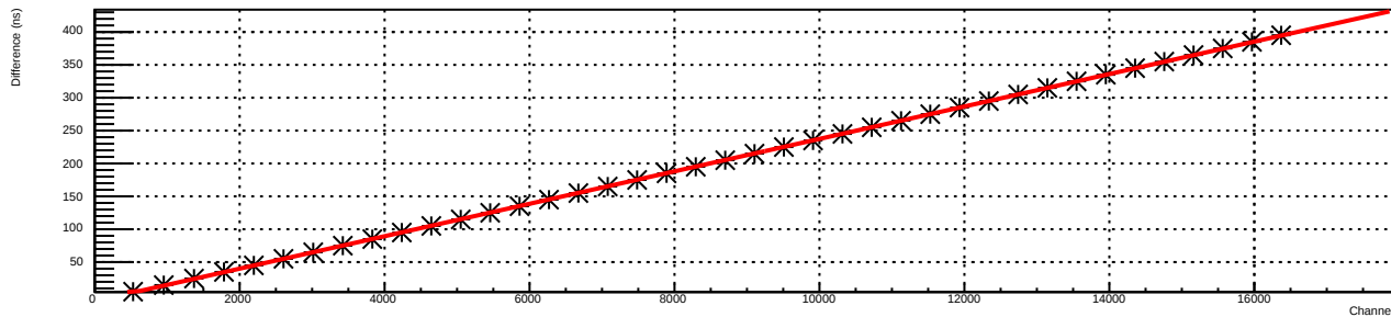
Histogram T_Si_Cats1
