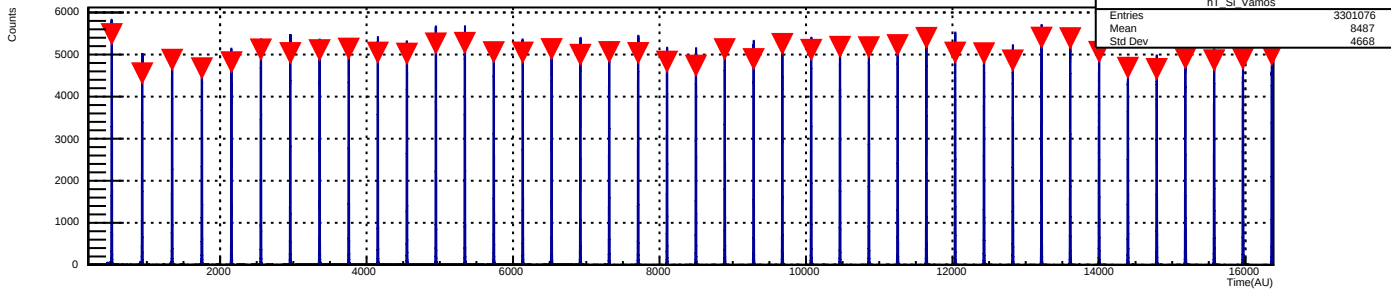
Histogram T_Si_Vamos
