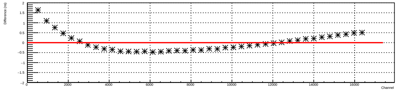
Histogram T_Si_Vamos
