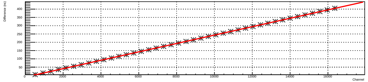
Histogram T_Si_Vamos
